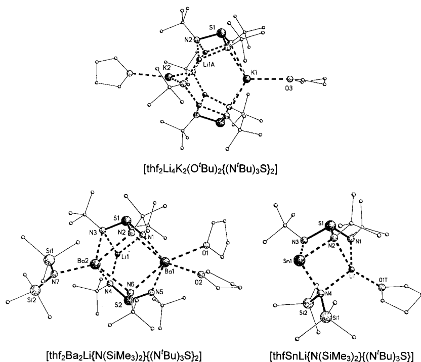
Fig. 6. Mixed metal complexes of \text{S}(\text{NR})_3^{2-} .
